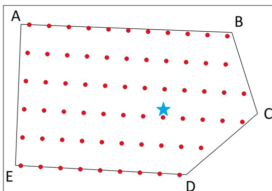
Illustration 2: Ensemble des points de grille AROME du domaine de l'étude (points rouges) et position de la bouée LIDAR prévue (étoile bleue)
