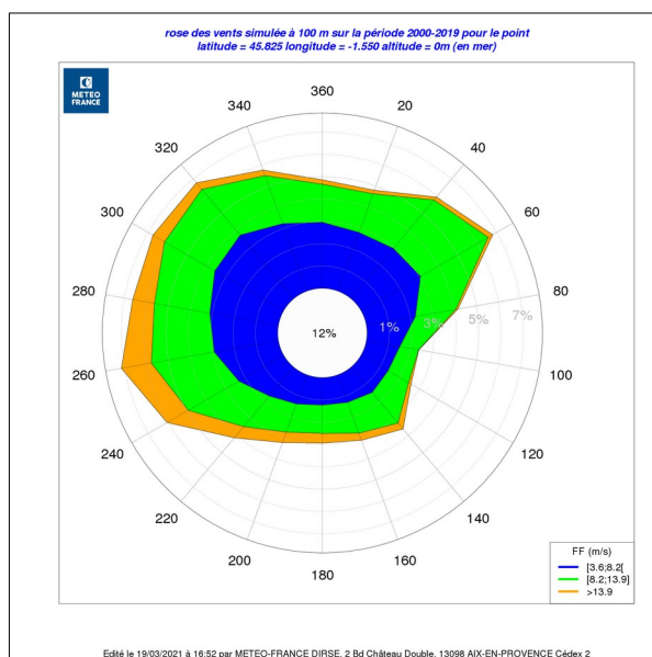
Illustration 3.2.1 : Rose des vents AROME 2000-2019 à 100 mètres de hauteur, au point le plus proche de la bouée
