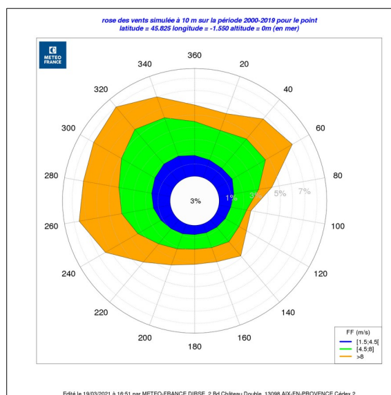
Illustration 3.4.1 : Rose des vents AROME 2000-2019 à 10 mètres de hauteur au point le plus proche la bouée
